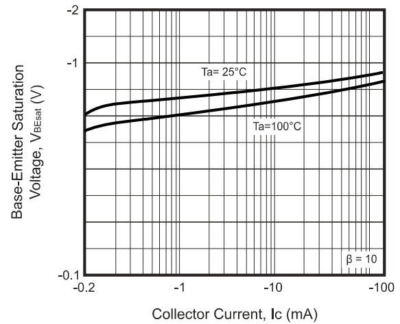
Fig.4 - V_{BEsat} - I_c
