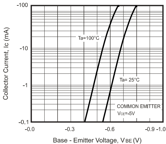
Fig.5 - V_{BE} - I_c
