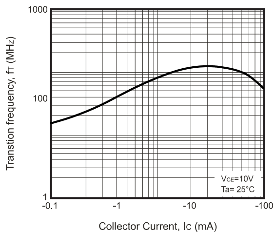
Fig.7 - f_T - I_c
