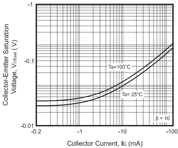
Fig.3 - V_{CEsat} - I_c
